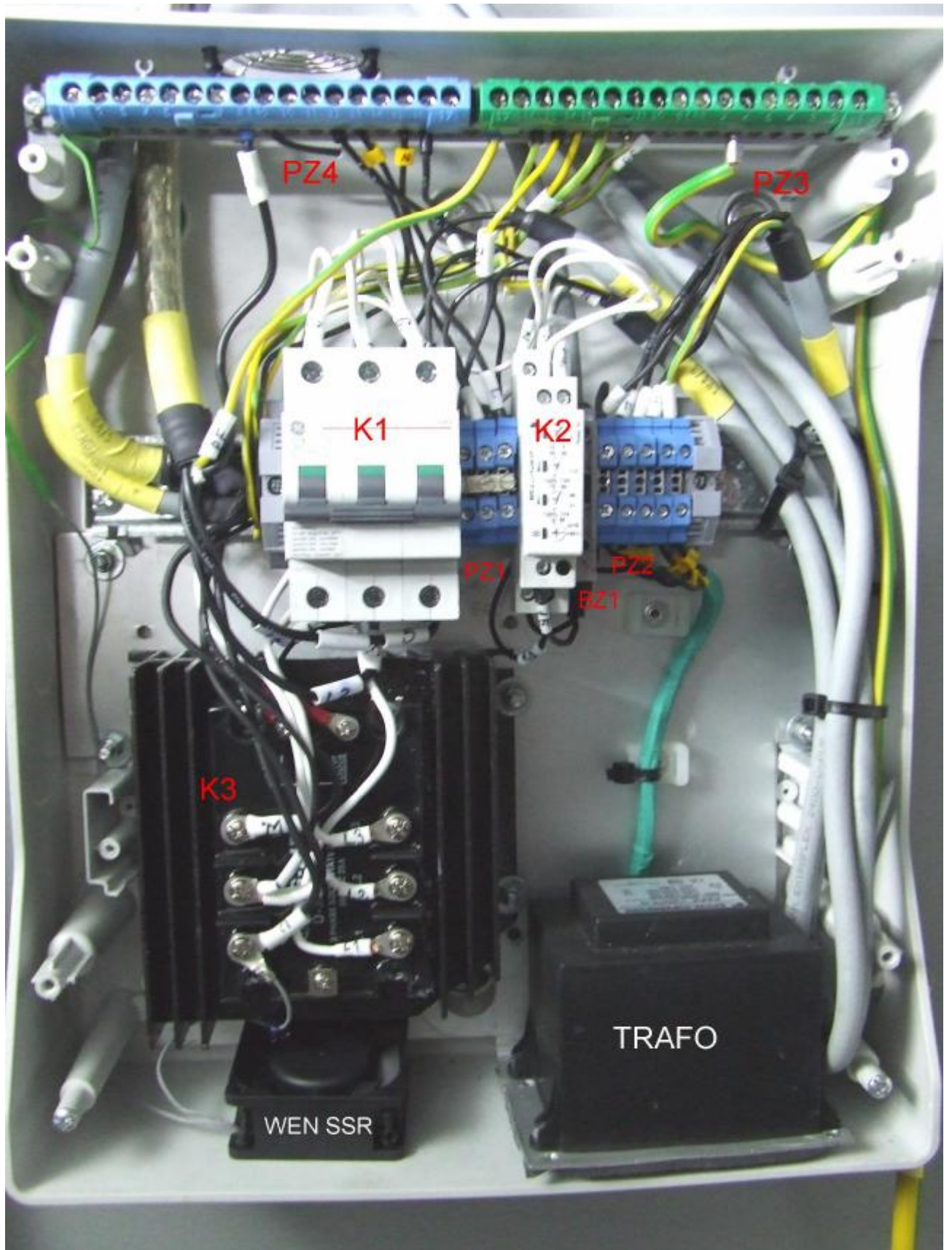
Rys 5 Widok wnętrza rozdzielni
