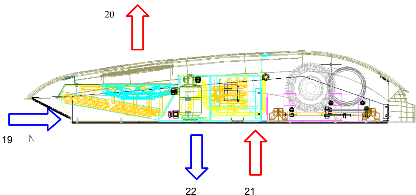
Rys. 4 Działanie klimatyzatora
